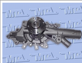
BOMBA DE AGUA Clase G 270 2.7 CDI (2001-->) Sprinter 213 308 311 313 408 411 2.2 CDI (1999-->2006)
