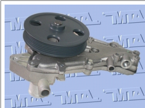
BOMBA DE AGUA Clio 1.6 C/AA Con Contracuerpo ( )
