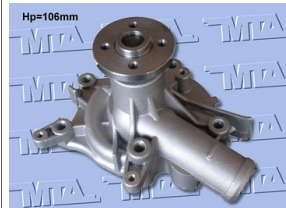
BOMBA DE AGUA Autoelevador 4G64 ( )
