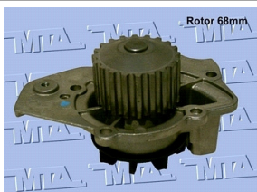
BOMBA DE AGUA Berlingo 1.9D (05.1998-->) Berlingo Multispace 1.9D (05.1998-->11.2010) Sin Solapa; Turbina 1201-60/62 68mm
